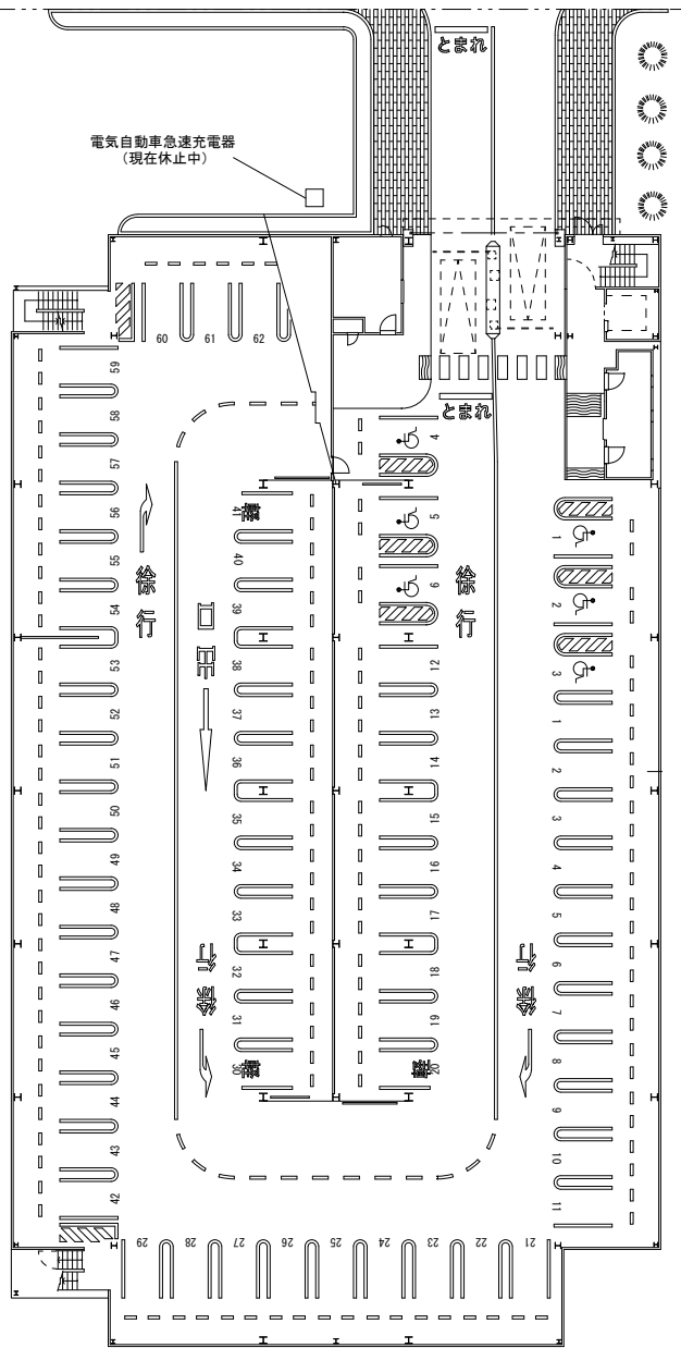
1階平面図
