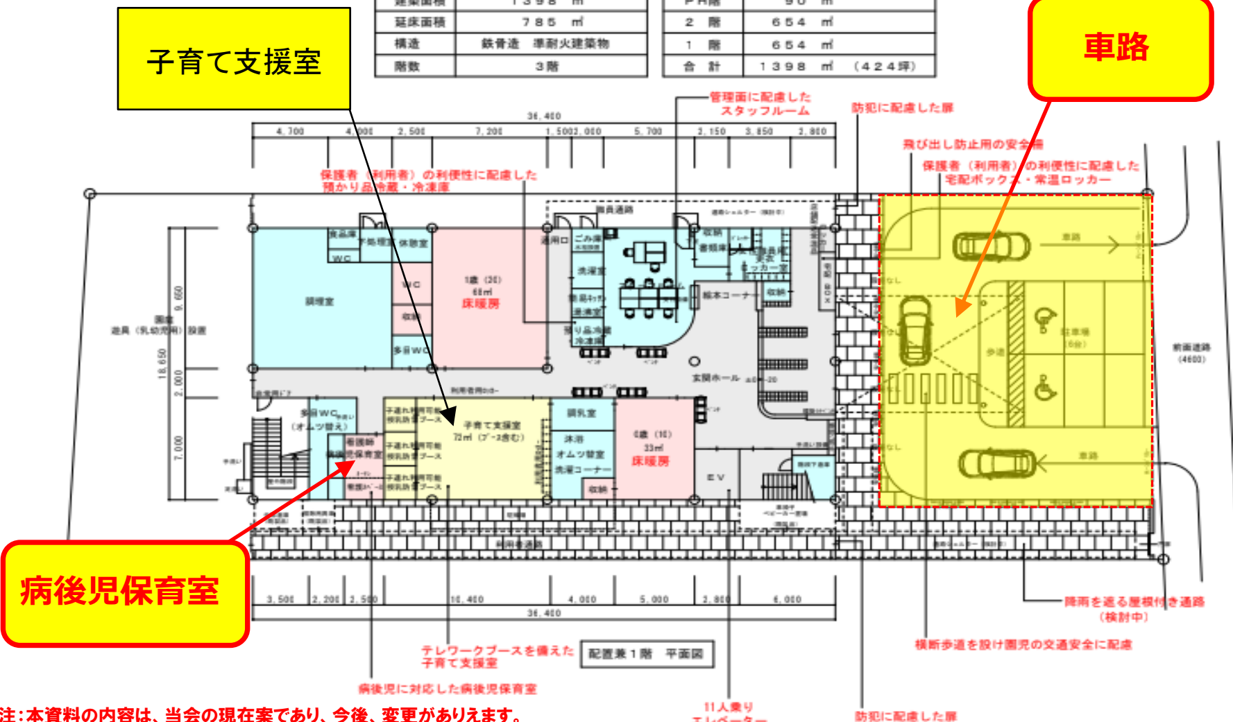
計画配置図兼1階平面図
