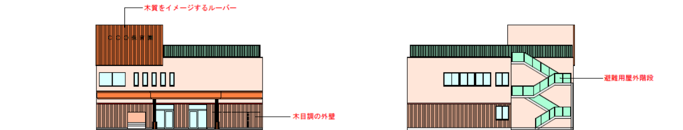
北 立面図
