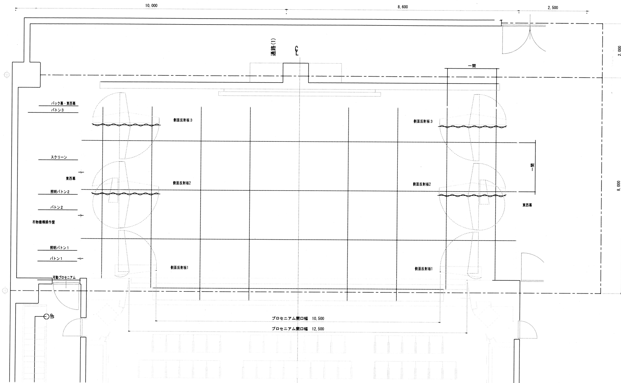
配置平面図
