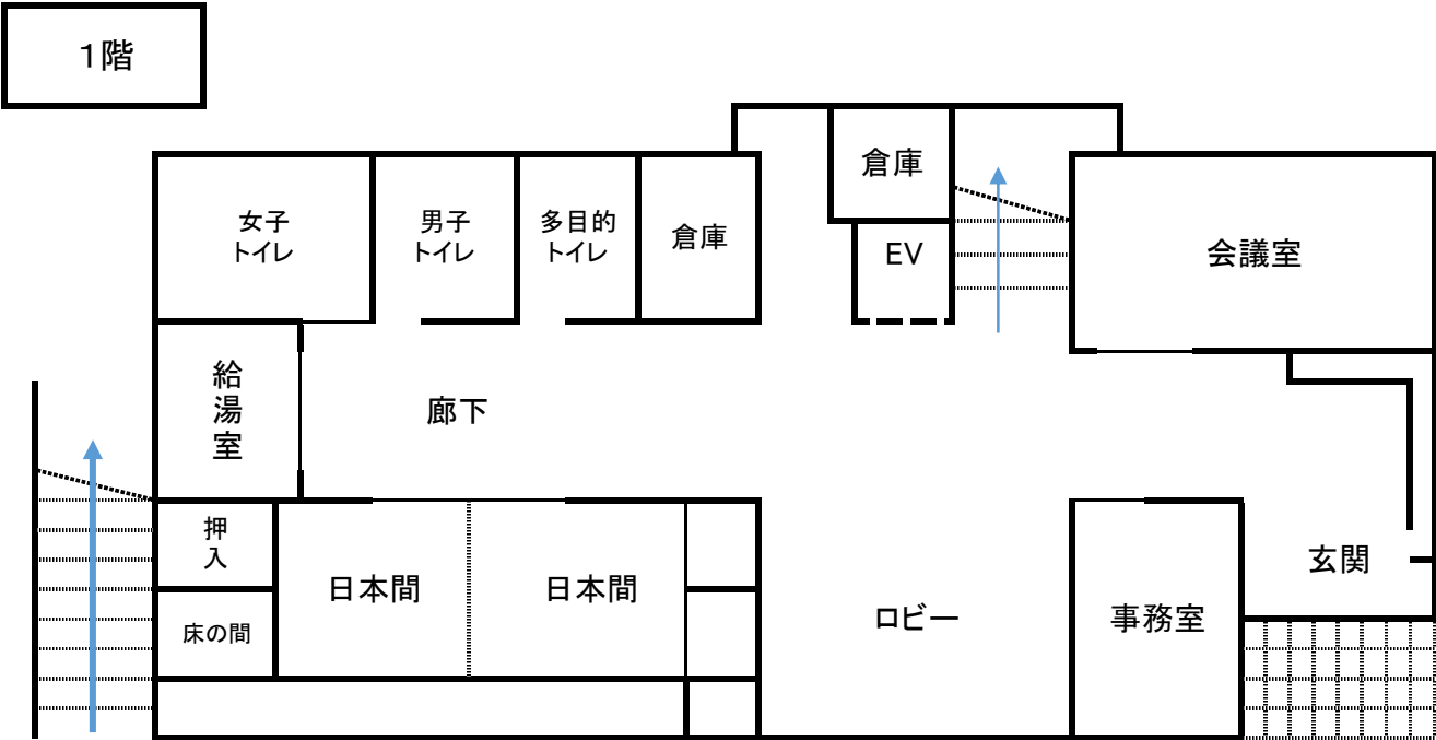
精義まちづくり拠点施設 平面図
