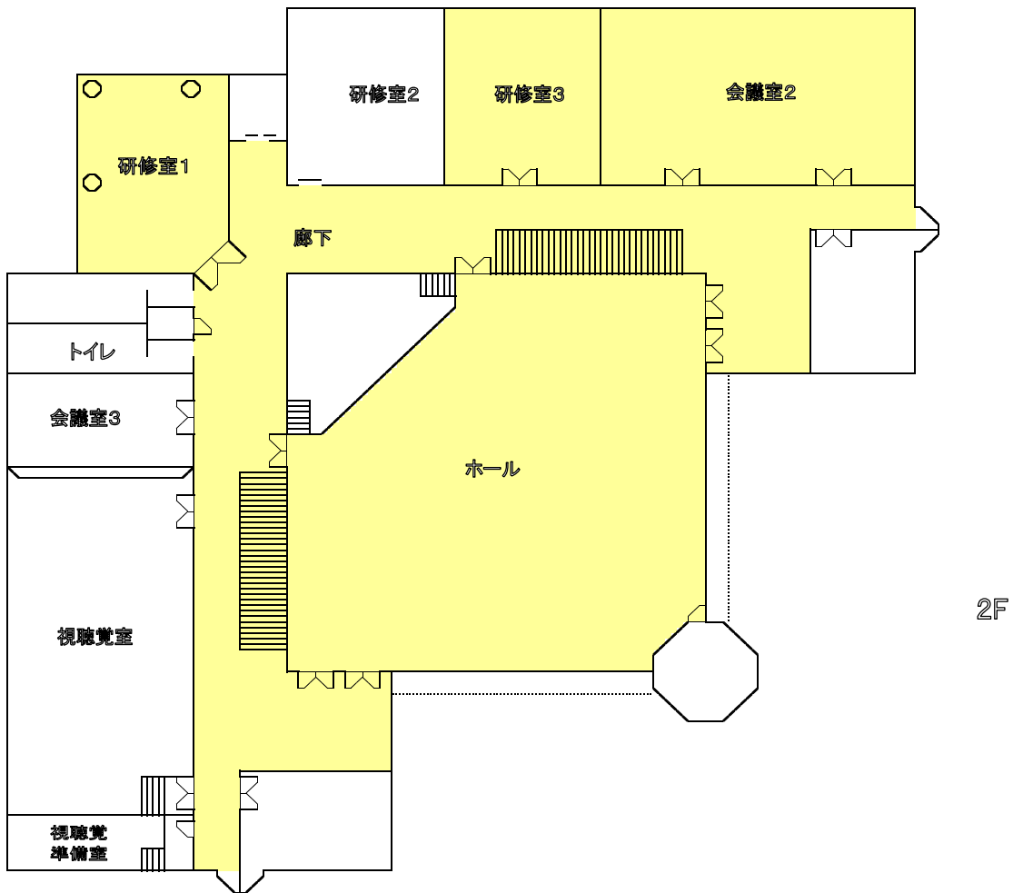
【図面】長島まちづくり拠点施設
