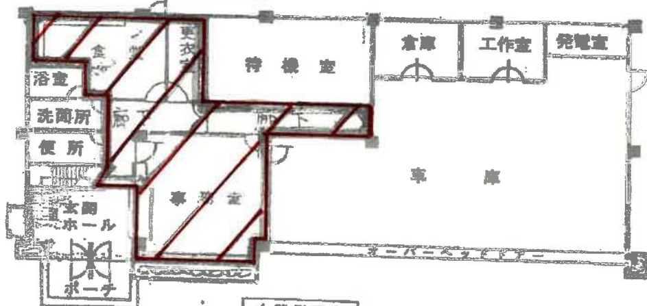
1階平面図
