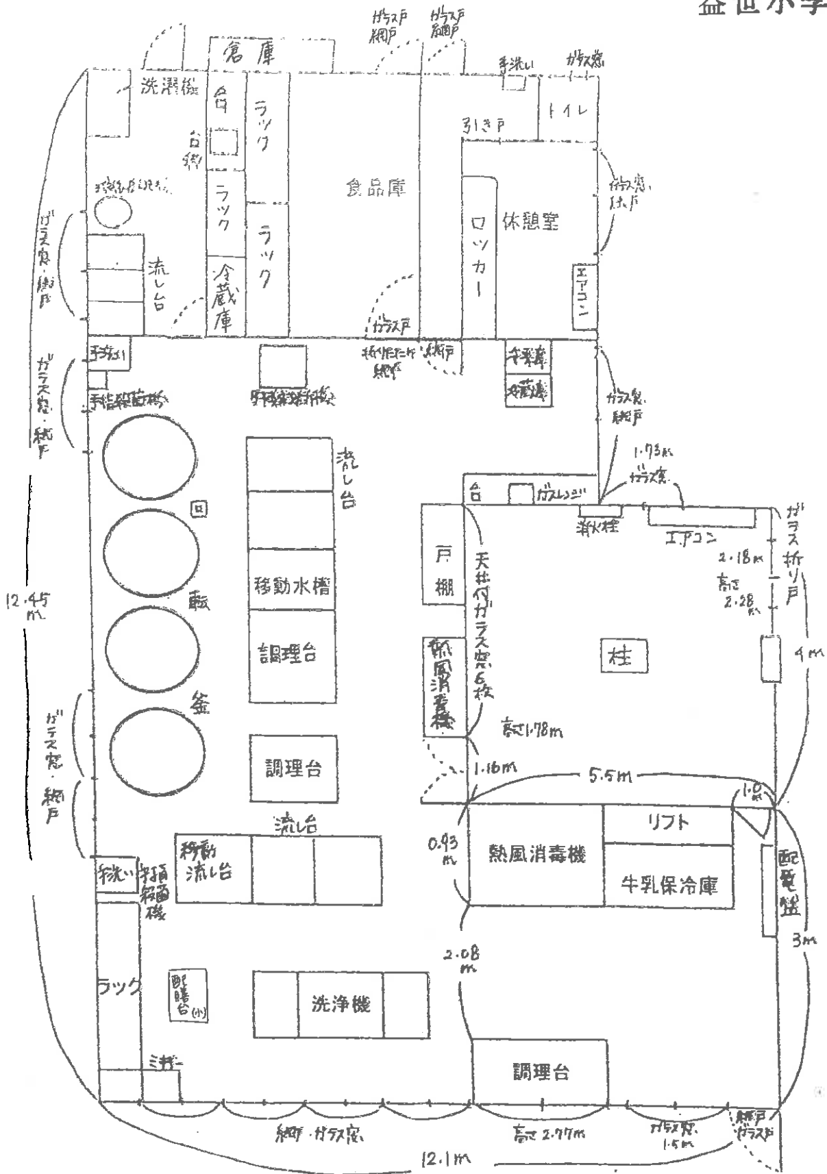
桑名市立益世小学校 給食室配置図
